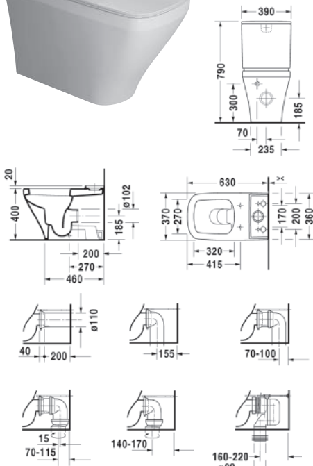
toilet 215509 vario outlet
