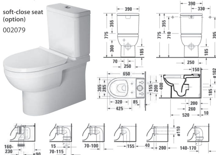
toilet 218209 vario outlet, rimless
