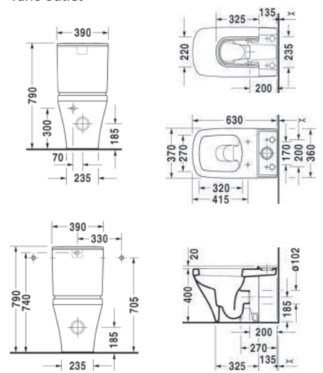
toilet 216209 vario outlet
