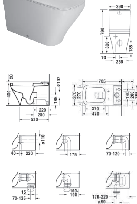
toilet 215609 vario outlet
